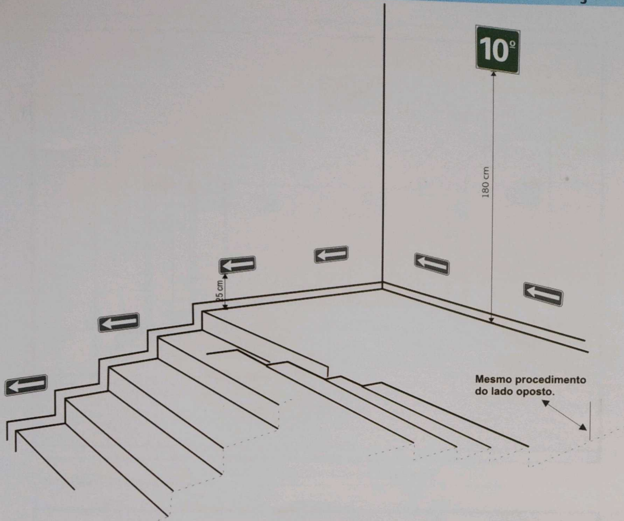
Sinalização complementar. Exemplo de rodapé
