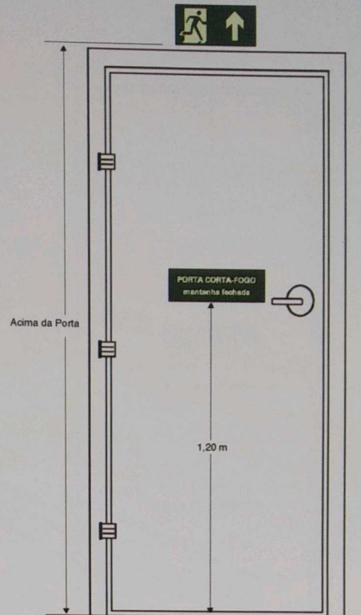
Sinalização de porta corta-fogo(vista da escada)
