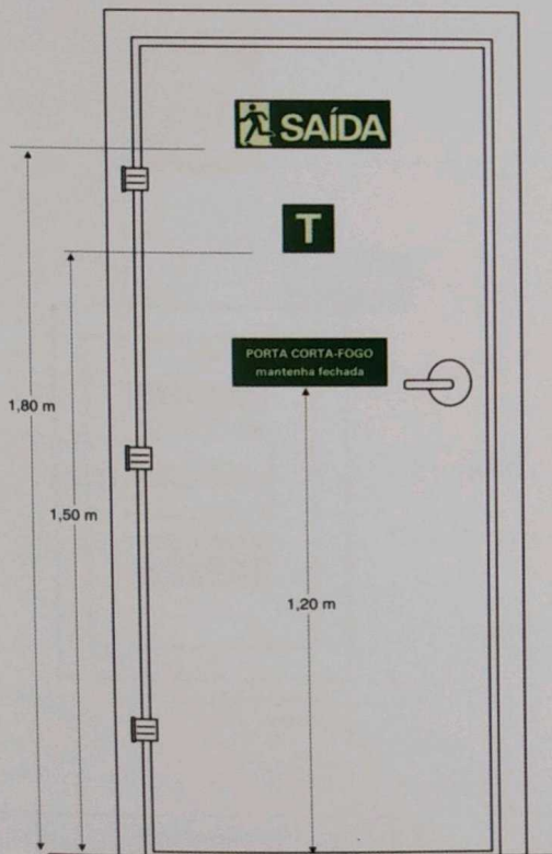
Sinalização de porta corta-fogo
